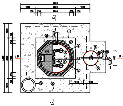
PŮDORYSNÝ REZ : A - A
