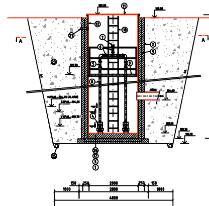
REZ : C-C
